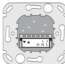
Несущая рамка Chronis Uno/Uno L вид сзади
